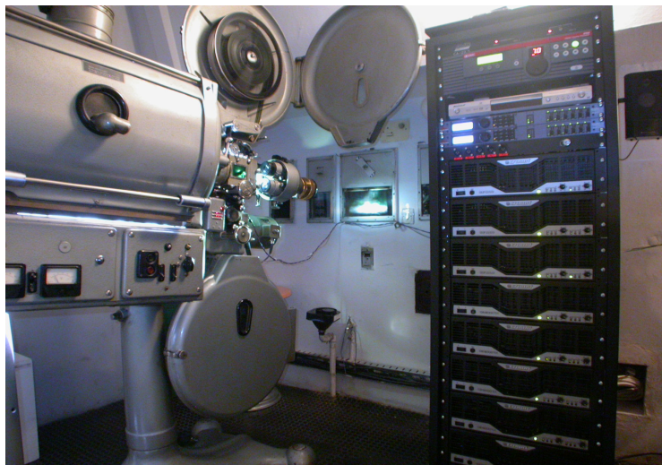
Slika 2 – Kino kabina bioskopa KCB
